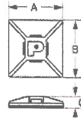
ABMM-A(-AT) (2個並び)
