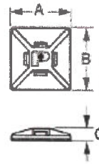
ABM1M-A(-AT) (4個並び)
