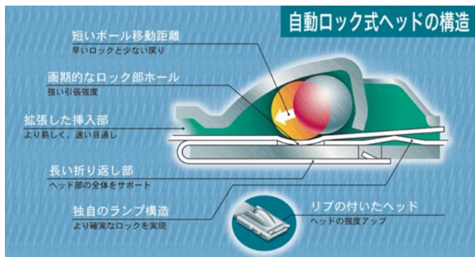
〈自動ロック式ヘッドの構造〉
